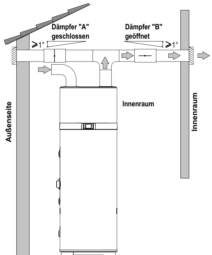
Abb. 14 - Beispiel der Installation im Sommer
