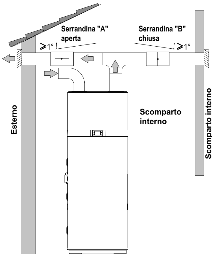
fig. 15- Esempio di installazione nel periodo invernale
