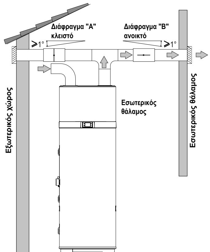
εικ. 14- Παράδειγμα εγκατάστασης στην καλοκαιρινή περίοδο
