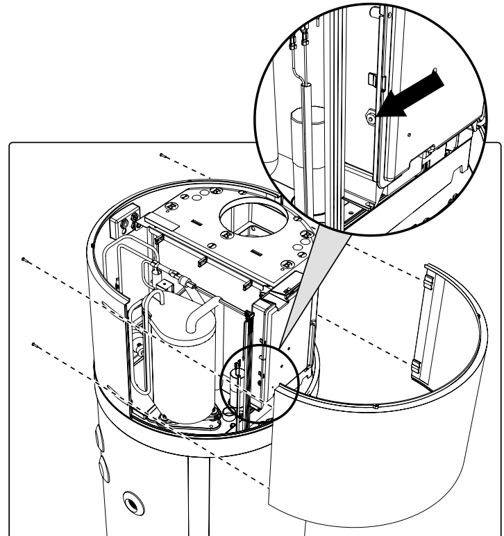
afb. 30- Verwijdering frontpaneel
