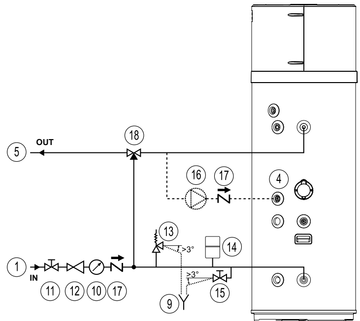
Abb. 17 Beispiel für das Wassernetz
