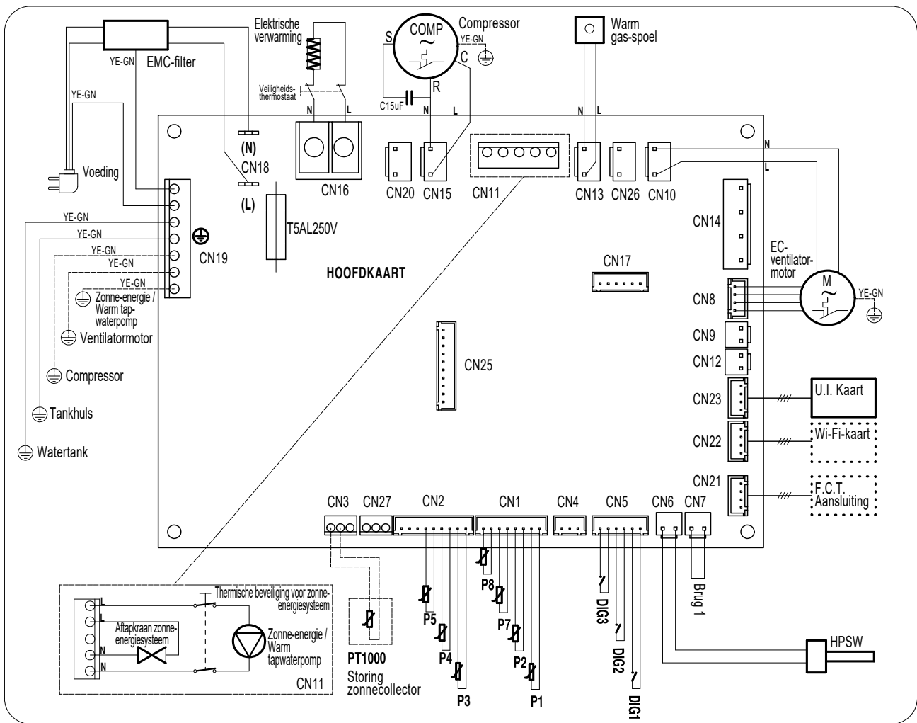
afb. 26- Bedradingschema van de apparatuur
