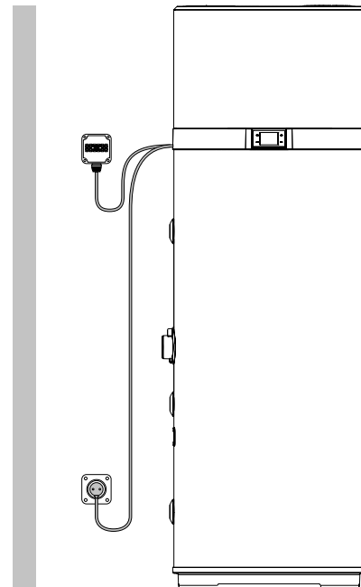
rys. 24- Przykład połączenia dodatkowego
