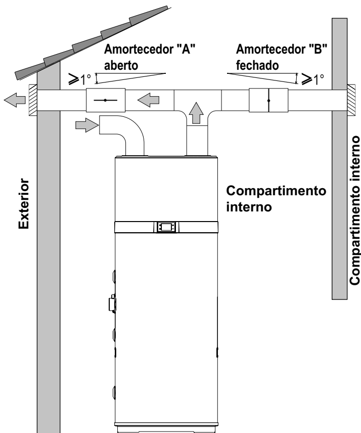
fig. 15- Exemplo de instalação no período do inverno
