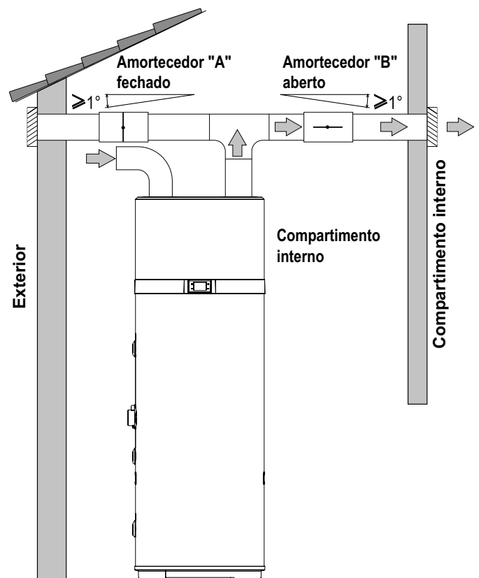
fig. 14- Exemplo de instalação no período do verão
