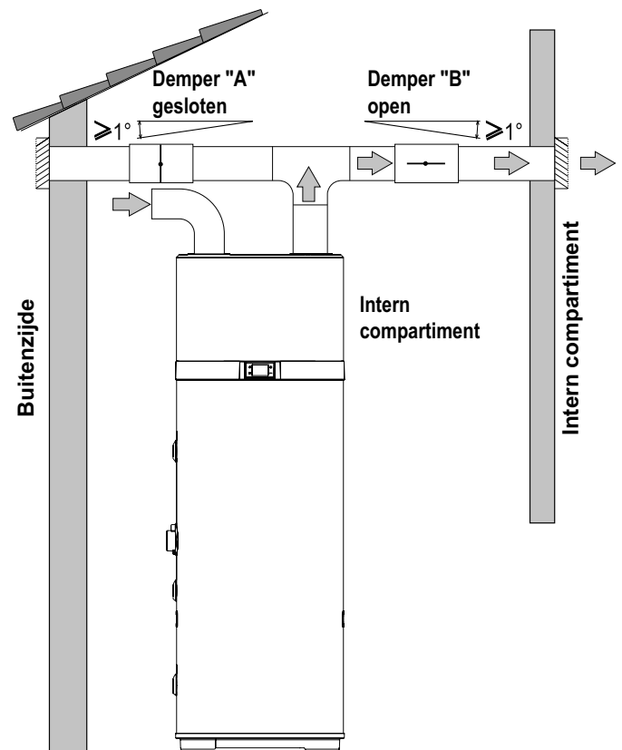
afb. 14- Voorbeeld van installatie in de zomerperiode
