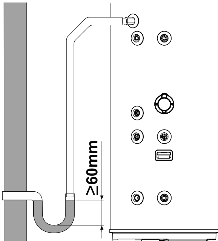
fig. 18- Exempel på kondensatdräneringsanslutning via ett lås
