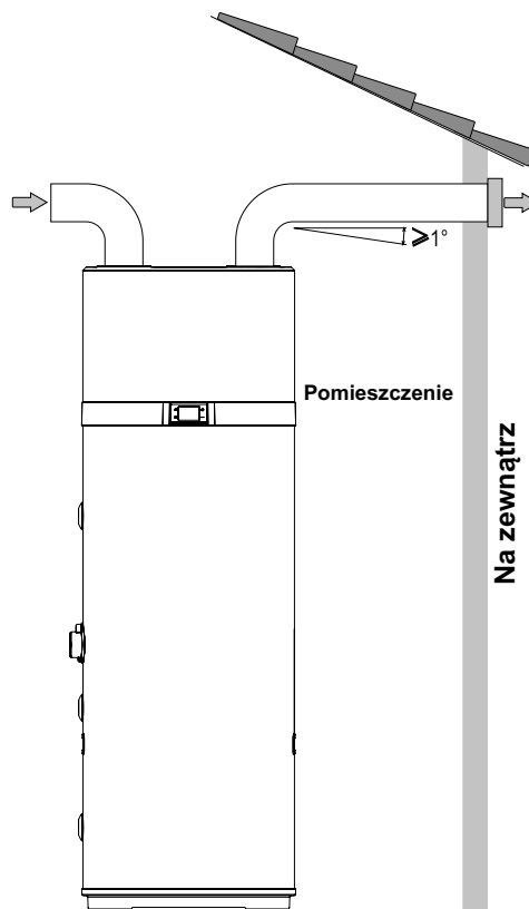
rys. 12- Przykładowe podłączenie wylotu powietrza
