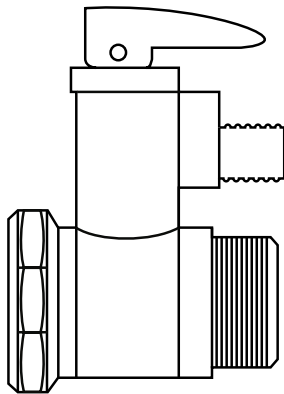
fig. 49 - Válvula de seguridad 0.7 MPa (7 bar)
