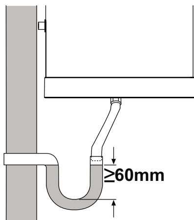
fig. 52 - Exemplo de ligação da drenagem da condensação com sifão
