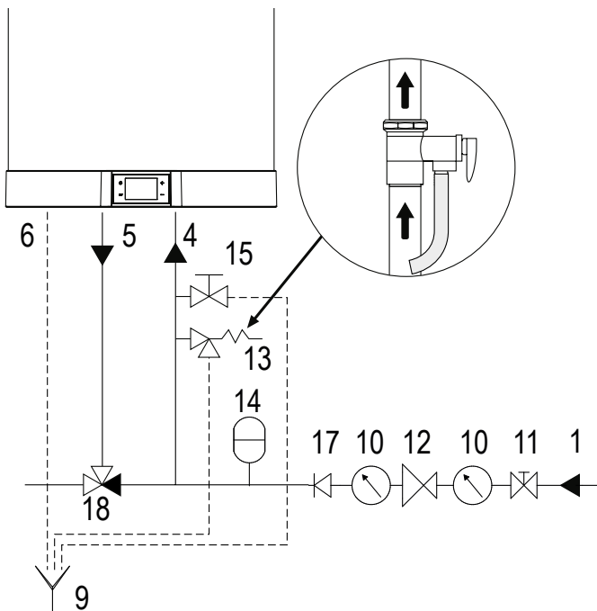
fig. 50 - Exemple installation hydraulique
