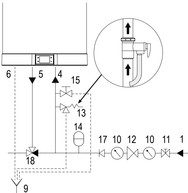
fig. 50 - Exemplo de sistema de água
