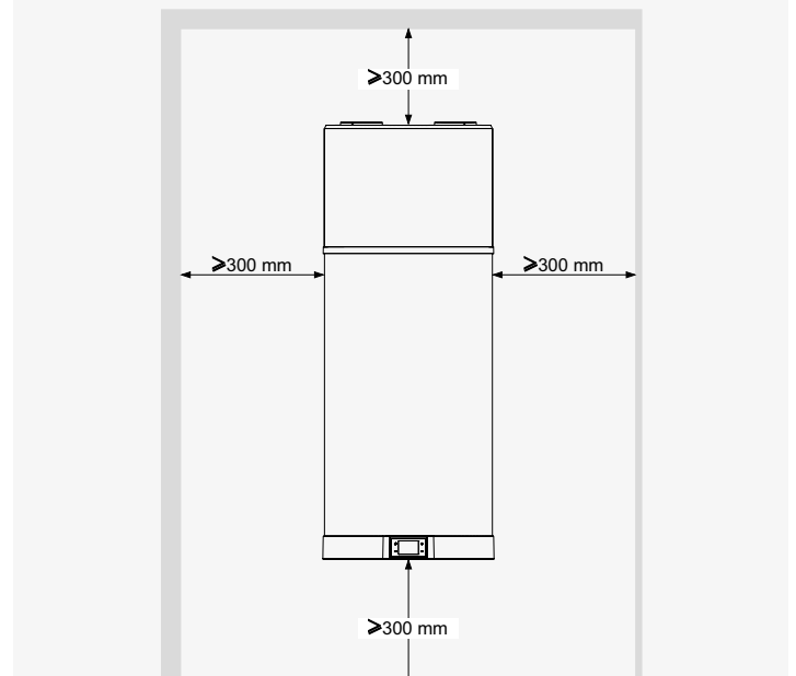
fig. 43 - Espaços mínimos
