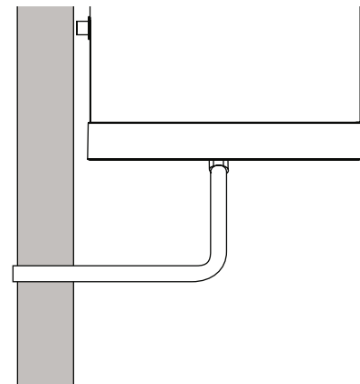
fig. 51 - Exemples de raccordement de l'évacuation des condensats sans siphon
