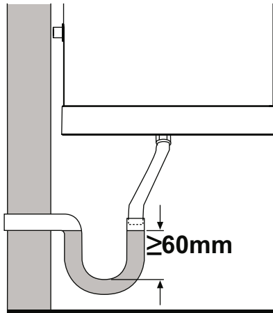
fig. 52 - Ejemplo de conexión del drenaje de condensado con sifón
