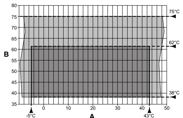
fig. 42 - Graphique
