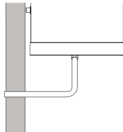
fig. 51 - Exemplo de ligação da drenagem da condensação sem sifão
