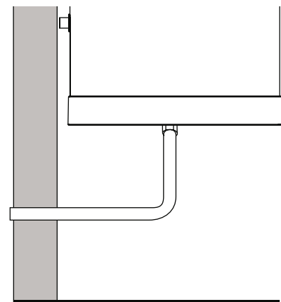
fig. 51 - Ejemplo de conexión del drenaje de condensado sin sifón
