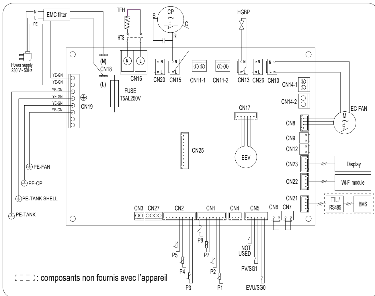
fig. 57 - Schéma de câblage de l'équipement
