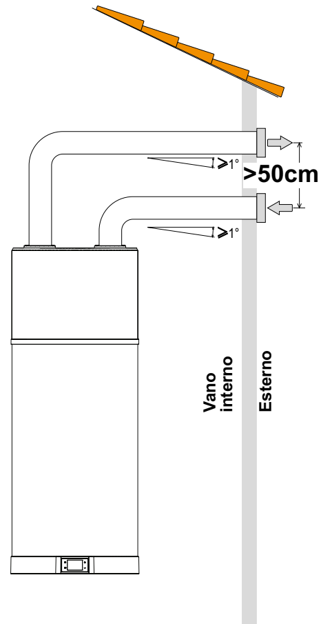
fig. 47 - Exemple de raccordement de l'échappement de l'air
