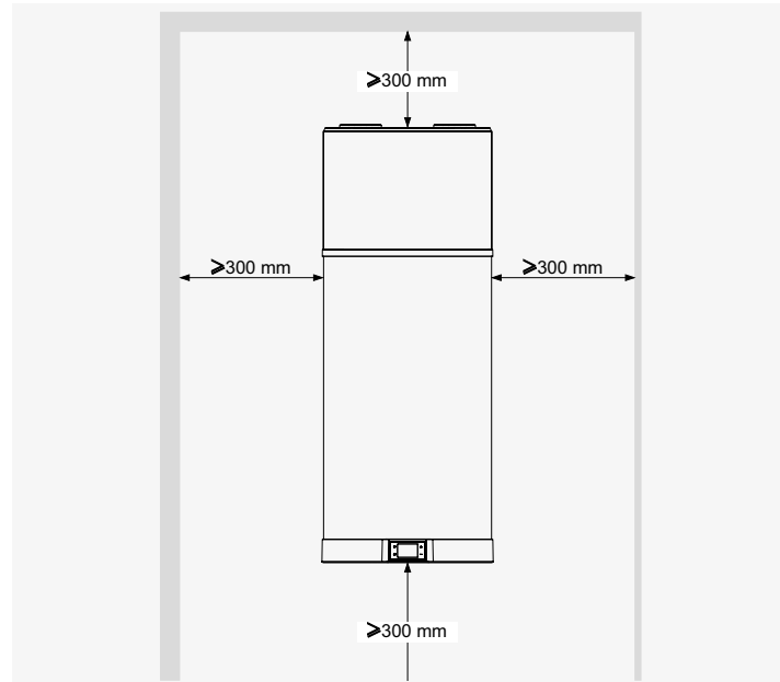
fig. 43 - Espaces minimum
