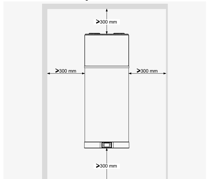
fig. 43 - Espacios mínimos
