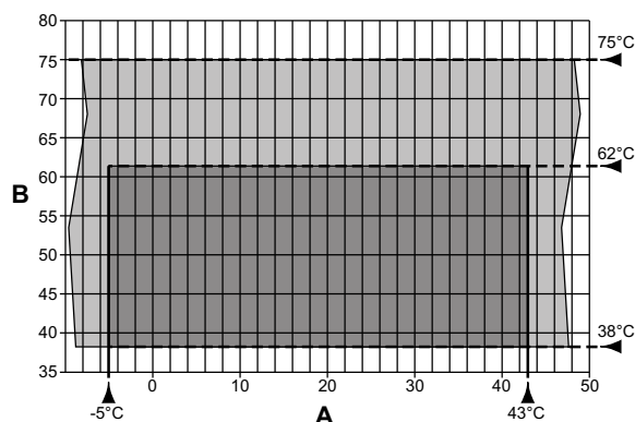
fig. 42 - Gráfico
