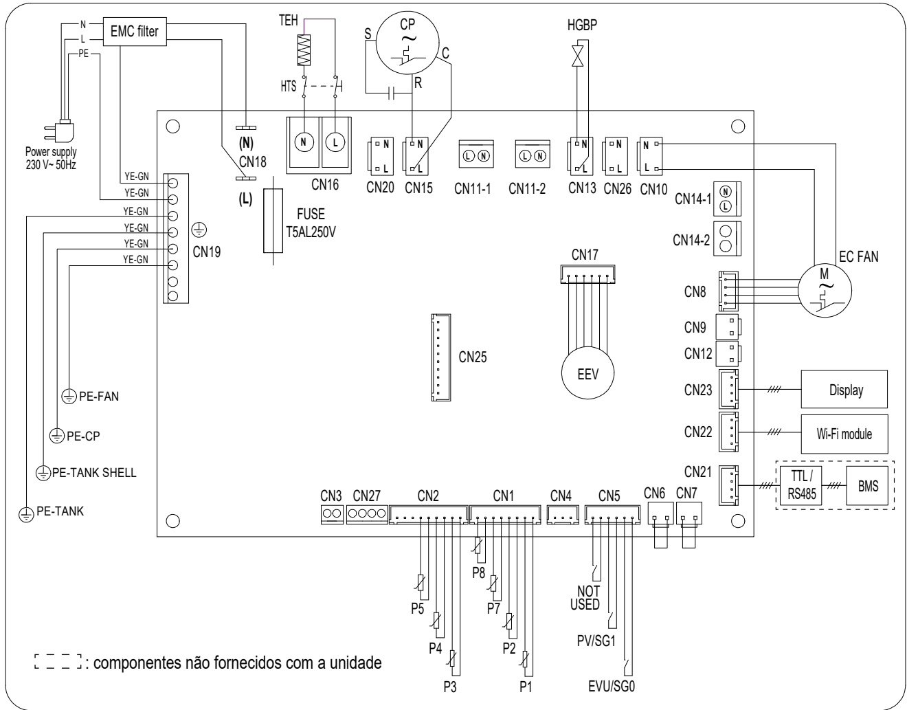
fig. 57 - Esquema elétrico do equipamento
