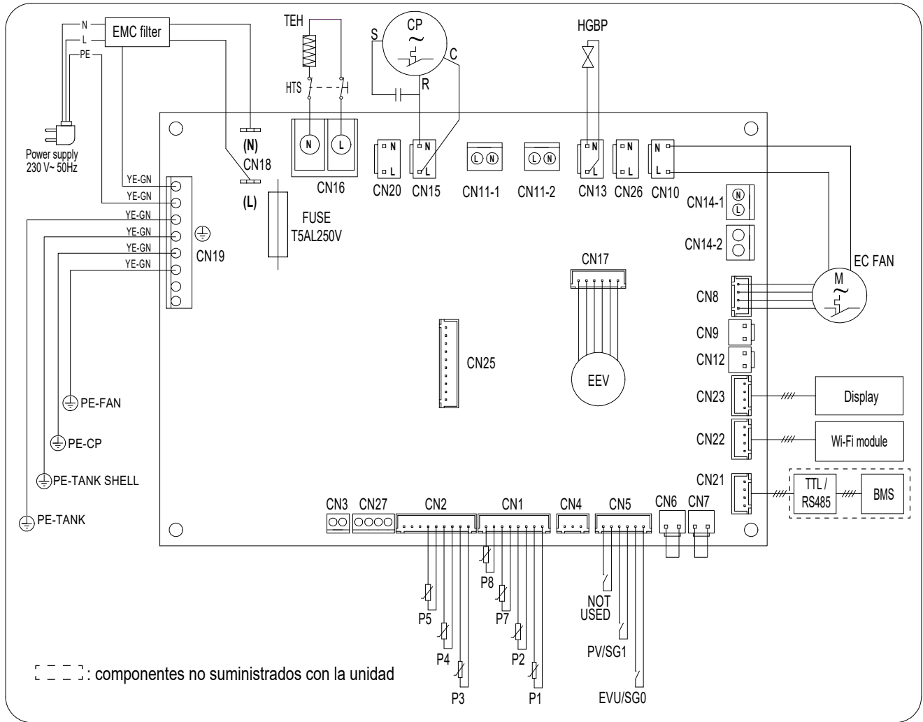
fig. 57 - Diagrama de cableado del equipo.
