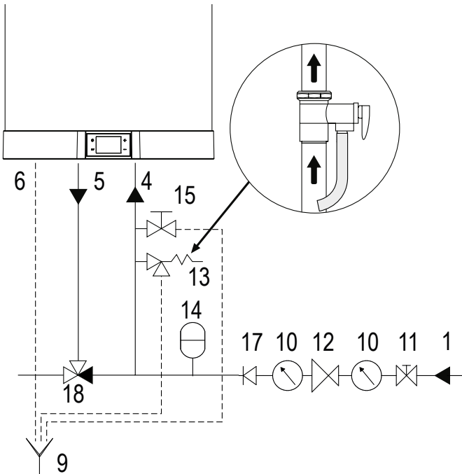
fig. 50 - Ejemplo sistema hidrico
